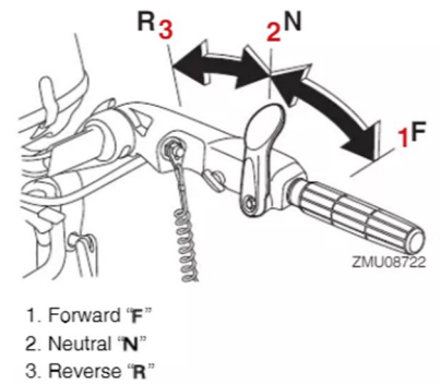
Obr.6 řazení 1:vpřed, 2:neutral, 3:vzad
