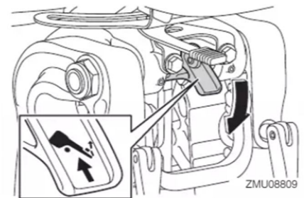
Obr.9 páka pro zvedání motoru
